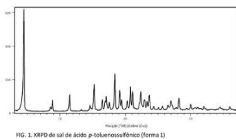
FIG. 1. XRPD de sal de ácido p-toluenossulfônico (forma 1)
