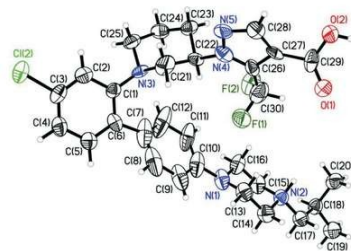
Figura 1: Ortep-Plot (50%) com esquema de rotulagem (sem desordem), exemplo 4
