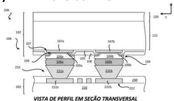
VISTA DE PERFIL EM SEÇÃO TRANSVERSAL
