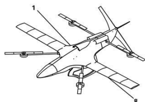
Figura 1 (1) VANT e (8) Sistema de Pulverização
