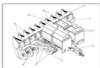
Figura 1 – vista isométria
