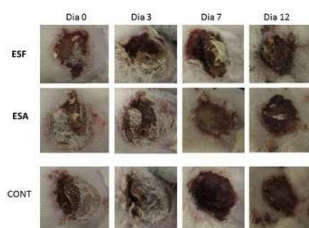
Figura 1. Evolução da cicatrização das lesões induzidas em ratos Wistar nos momentos: 0h (anterior aos tratamentos), 3, 7 e 12 dias após o início da aplicação dos tratamentos.
