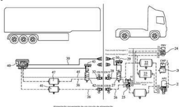
Arbitragem apresentada de um circuito de suspensão
