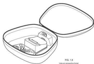
FIG. 1.8 Vista em perspectiva frontal
