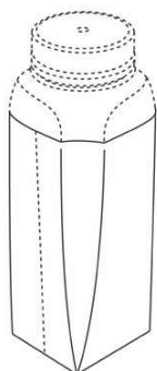
FIG. 2.1 Vista em perspectiva frontal, superior
