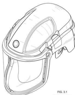
FIG. 3.1 Vista em perspectiva frontal, superior
