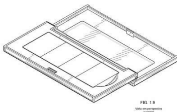
FIG. 1.9 Vista em perspectiva superior
